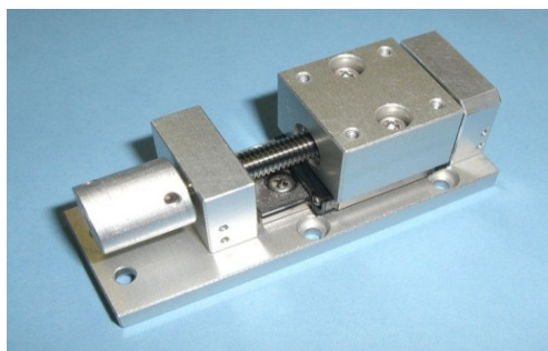
②送りねじ:TMG5(精密研削ねじ)使用
