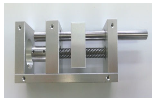
④送りねじ:TMH8-10(ハイリードねじ)使用
